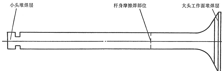
图 1 气门示意图
